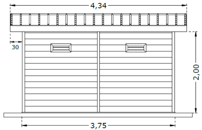
Ansicht hinten / rear view
