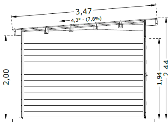
Schnitt / section
