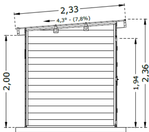
Schnitt / section
