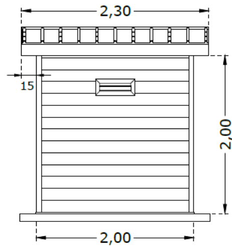
Ansicht hinten / back view
